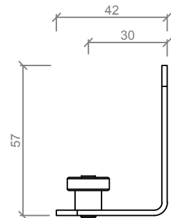
ROLLER GUIDE
