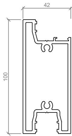
ASL 670 100mm TRANSOM
