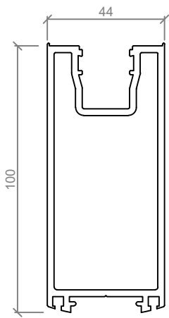
ASL 660 100mm LOCKSET STILE
