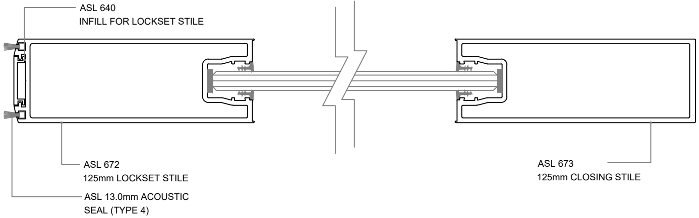
HINGED DOOR
